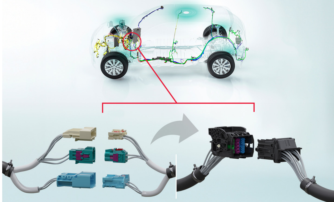
複数のコネクタを単一のMX-DaSHモジュラーインターフェースに置き換え、ハーネス設計の複雑さを軽減
